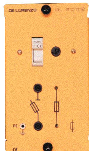
DL 2101T12 PORTAFUSIBLES Aislador con fusibles de cartucho 2 A 500 V. Portafusible con fusible miniatura 2 A, 250 V.
