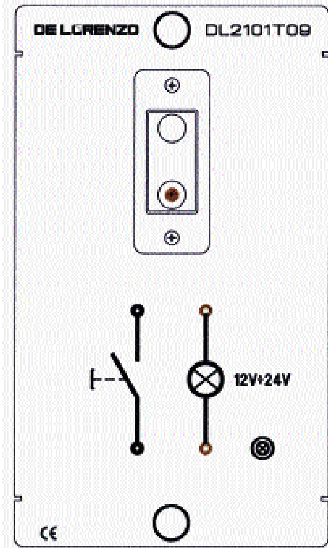
DL 2101T09 PULSANTE LUMINOSO Interruptor unipolar 250 Vca, 10 A. Completo con lámpara piloto 24 Vca.
