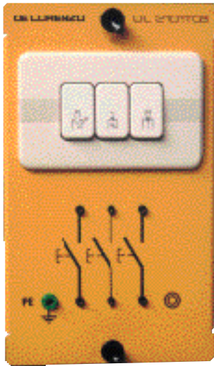
DL 2101T08 PULSADOR CAMARERA/CAMARERO Tres interruptores unipolares 250 Vca, 10 A.
