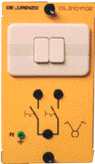
DL 2101T02 CONMUTADOR Doble interruptor unipolar 250 Vca, 10 A.
