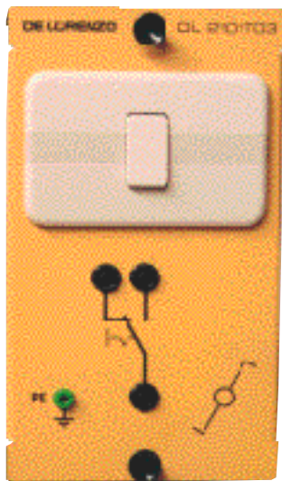
DL 2101T03 DESVIADOR Interruptor bidireccional 250 Vca, 10 A.
