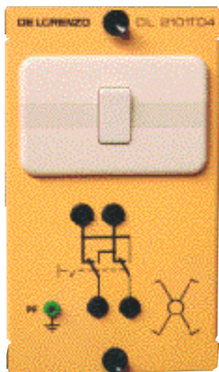
DL 2101T04 INVERSOR Interruptor intermedio 250 Vca, 10 A.
